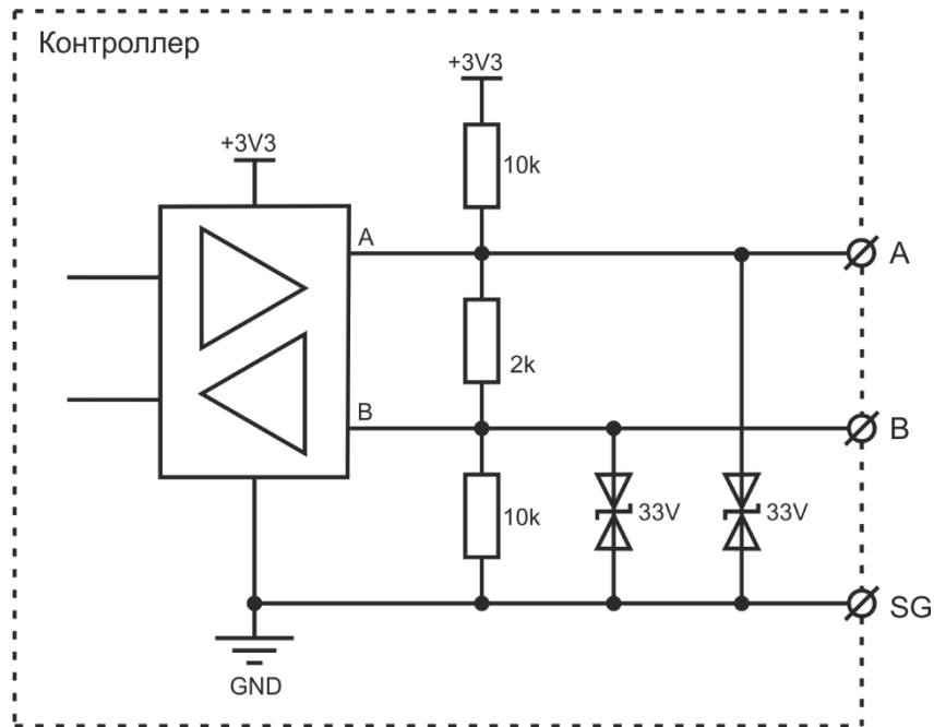
Рисунок 6.1 - Порт RS-485
